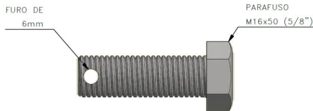
Figura 2 – Parafuso com Rosca completa
