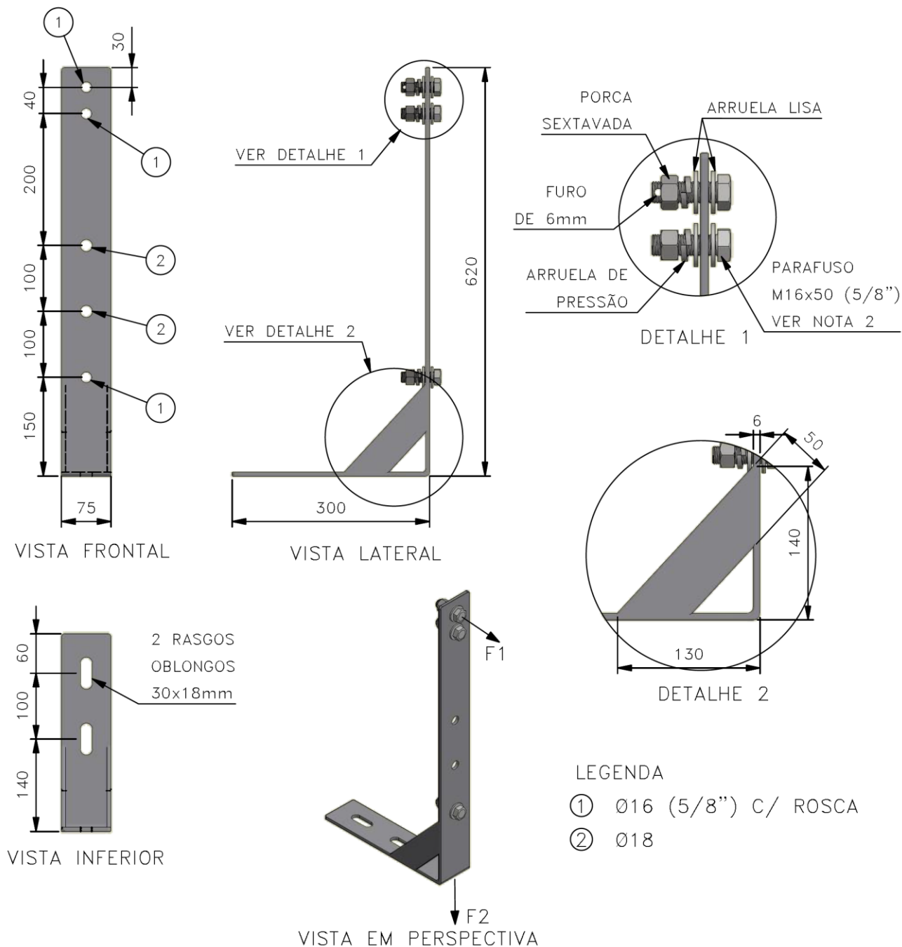
Figura 1 – Suporte L para Fixação de Concentrador em Rede DAT
